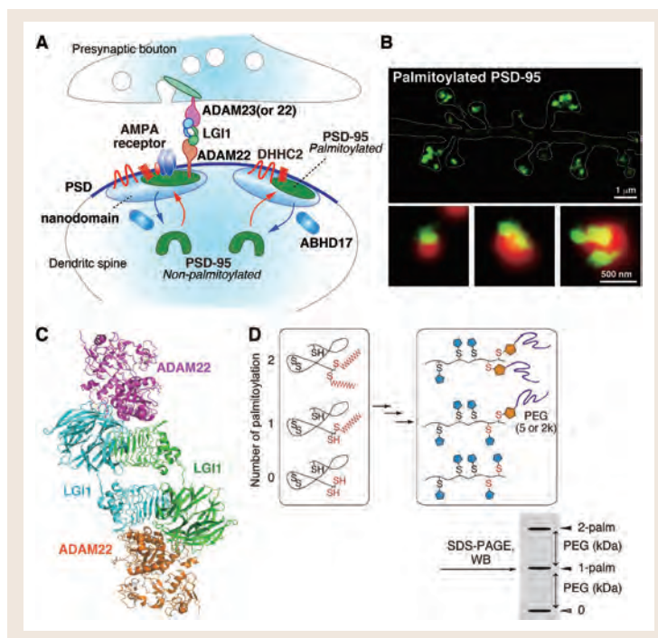
図 (A) 独自に発見した AMPA 受容体制御分子：パルミトイル化酵素 DHHC、脱パルミトイル化酵素 ABHD17 とてんかん関連リガンド・受容体 LGI1・ADAM22、そして、パルミトイル化 PSD-95 で構成されるナノドメイン。(B) パルミトイル化 PSD-95 特異的プローブと超解像顕微鏡によるポストシナプスナノドメインの発見。(C) LGI1・ADAM22 複合体の X 線結晶構造。(D) パルミトイル化修飾率の定量的解析法。
