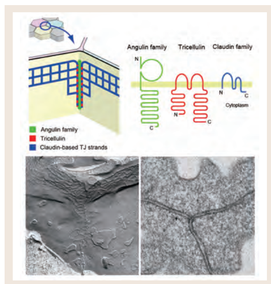
トリセルラータイトジャンクション分子構築と超微形態。
