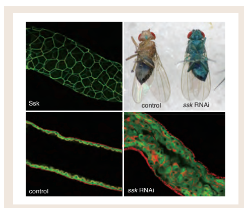
ショウジョウバエの腸管における細胞間結合スミースセプテートジャンクションの機能
