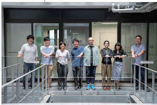
ヒト脳波ー TMS 同時計測実験を行い, 脳波ダイナミクスのデータ解析と数理モデル化により神経ダイナミクスの機能的役割の理解を目指します。
