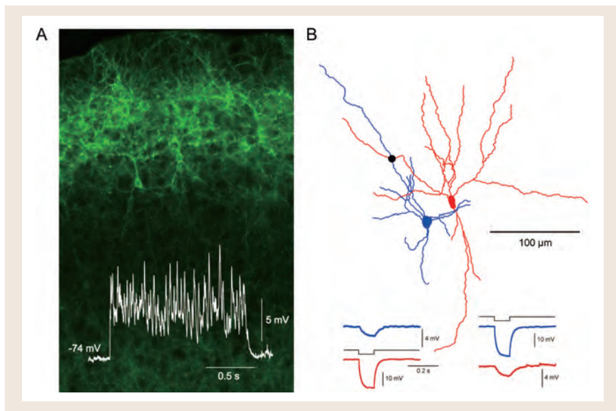
(A) 光刺激によって誘発される大脳皮質のネットワーク活動。2/3 層錐体細胞に選択的にチャネルロドプシン (Venus をタグ) を発現させ (写真), 5 層錐体細胞からホールセル記録をスライス標本において行った。光刺激中に膜電位のオシレーションが誘発された。
