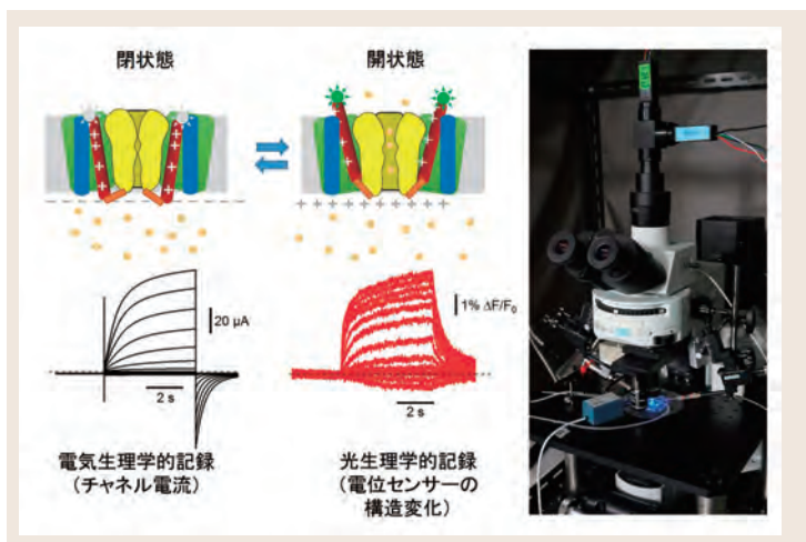
図1 アフリカツメガエル卵母細胞を用いた、膜電位固定下でのチャネル電流と蛍光強度の同時測定による、KCNQ1/ KCNE1 \text{K}^+ チャネル複合体の機能と動的構造変化の解析 (Nakajo and Kubo, Nature Commun (2014))
