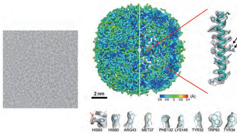
図2 アポフェリチンのクライオ電顕像 (左) と三次元再構成されたマップ (右)。
