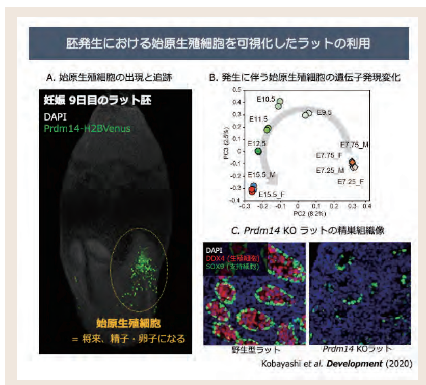
図1. 胚発生における始原生殖細胞 (PGC) を可視化した Prdm14-H2BVenus ラットの作製とその利用. A) H2BVenus 発現を指標に PGC を追跡し、PGC の出現時期と部位、その後の動態を明らかにした。B) 胚発生段階が異なる PGC のトランスクリプトーム解析 (8,966 遺伝子) から、発生段階 (E7.25 ~ E15.5) に応じた遺伝子発現の変化を明らかにした。F: 雌, M: 雄。C) Prdm14 KO ラット精巣を免疫組織染色したところ、ライディッヒ細胞やセルトリ細胞は観察されたが、生殖細胞はまったく認められなかった。
