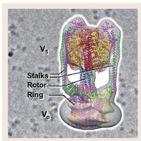
図2 クライオ電子顕微鏡により明らかになった腸球菌の V-ATPase の構造。背景はその電顕像。(Tsunoda et al. 2018)。
