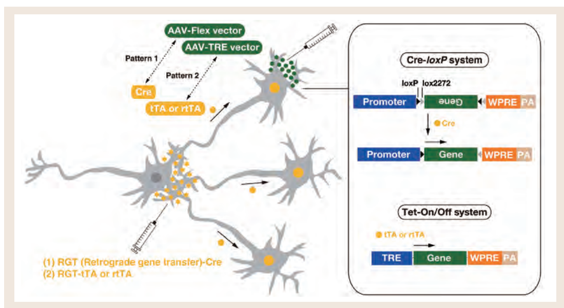
図1 ウィルスベクターを利用した脳内特定神経路への遺伝子導入。逆行性遺伝子導入 (RGT) ウィルスベクターとアデノ随伴ウィルス (AAV) ベクターを組み合わせた二重ベクターシステムを利用することによって、脳内の特定神経路でのみ目的遺伝子を発現誘導することが可能になります。各種ウィルスベクターは、共同研究として提供可能です。
